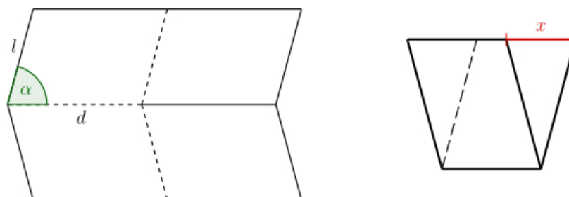
Obr. 7: Základná časť vzoru Miura v rozloženom a zloženom tvare
