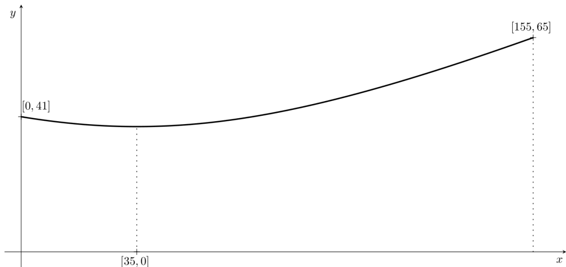
Figura 2: Sección transversal de una torre de refrigeración horizontal. La corona de la torre está situada a la izquierda y la base a la derecha.
