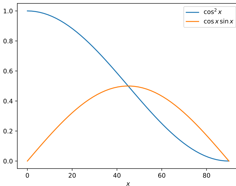
Obrázek 5: Průběh funkcí \cos^2 x a \cos x \sin x pro proměnnou x ve stupních. Tyto funkce udávají, v jakém poměru se rozdělí namáhání tyče na normálovou a smykovou složku.
