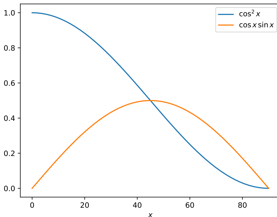
Obrázek 6: Průběh funkcí \cos^2 x a \cos x \sin x pro proměnnou x ve stupních. Tyto funkce udávají, v jakém poměru se rozdělí namáhání tyče na normálovou a smykovou složku.
