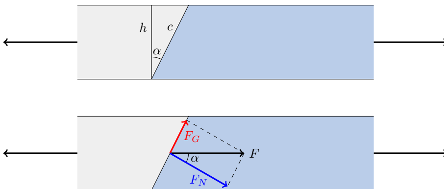
Obrázek 5: Šikmý spoj. V horní části trojúhelník pro výpočet délky strany spoje, v dolní části trojúhelník pro rozklad síly F do tečného a normálového směru.
