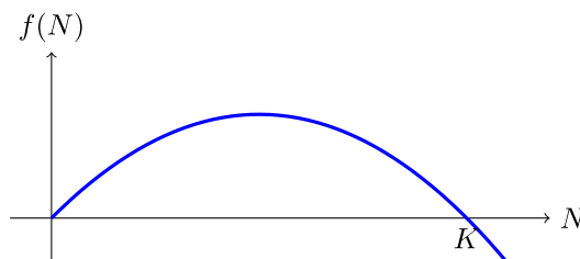
Figura 2: Tasa de crecimiento de la población en función del tamaño de la población.
