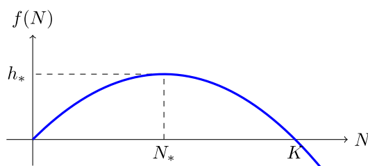
Figura 3: Tasa de crecimiento de la población en función del tamaño de la población, indicando la intensidad máxima posible de explotación h_* y el tamaño de población estable correspondiente N_* .
